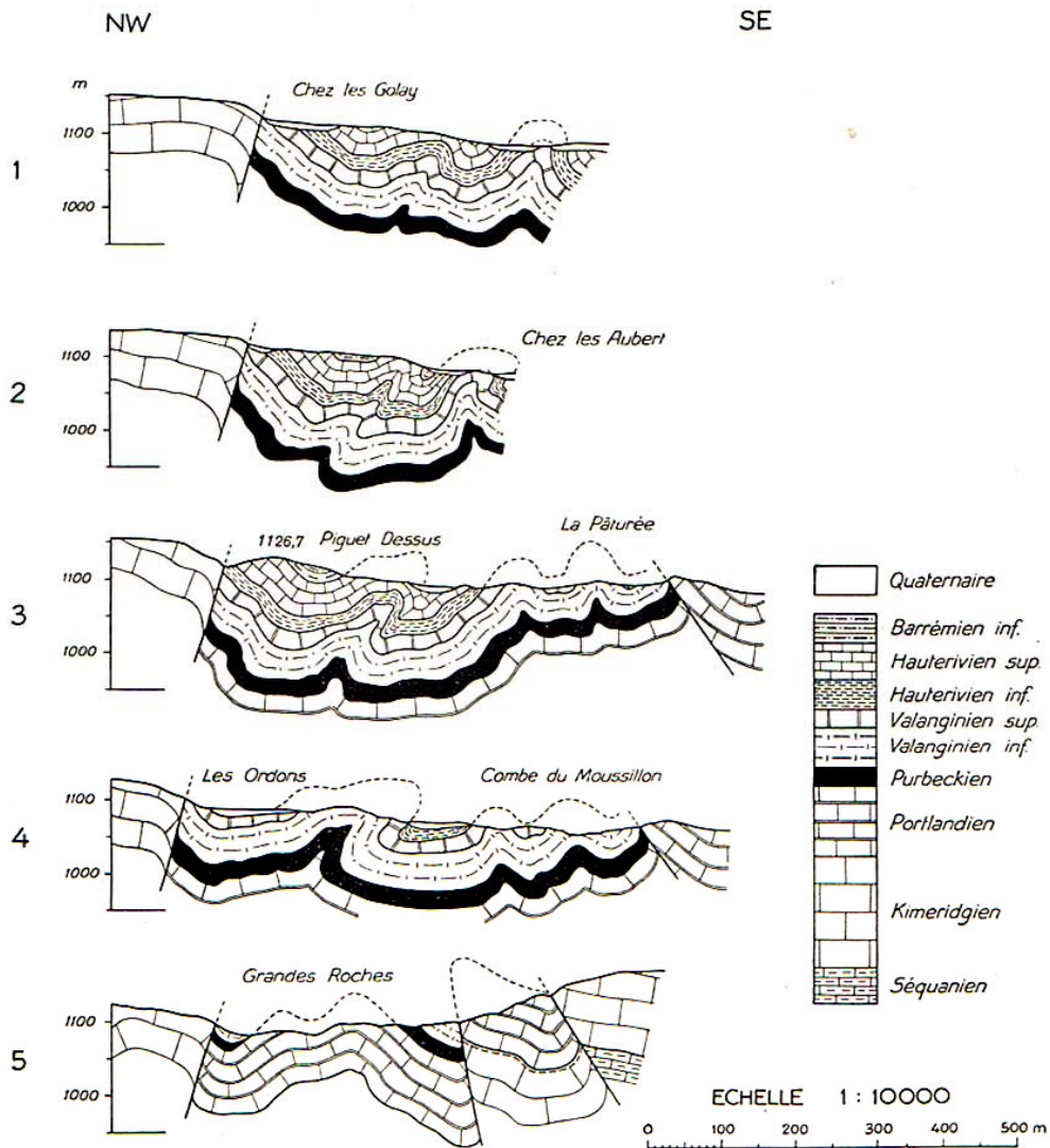
Fig. 20. Coupes tectoniques de la région des Pignet Dessus.
