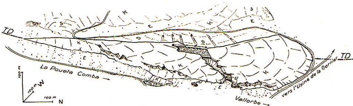
Fig. 26. Lambeau de recouvrement de la Dernier.
