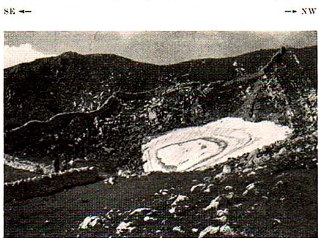
Fig. 32. Doline ou «creux à neige» près du sommet du Mont Tendre. Photographie prise au mois de juillet. Photo Aubert.
