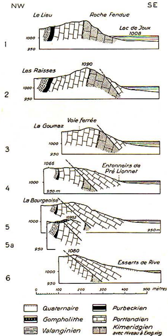
Fig. 17. Coupes géologiques de l'enjambement de Pré Lionnet.
