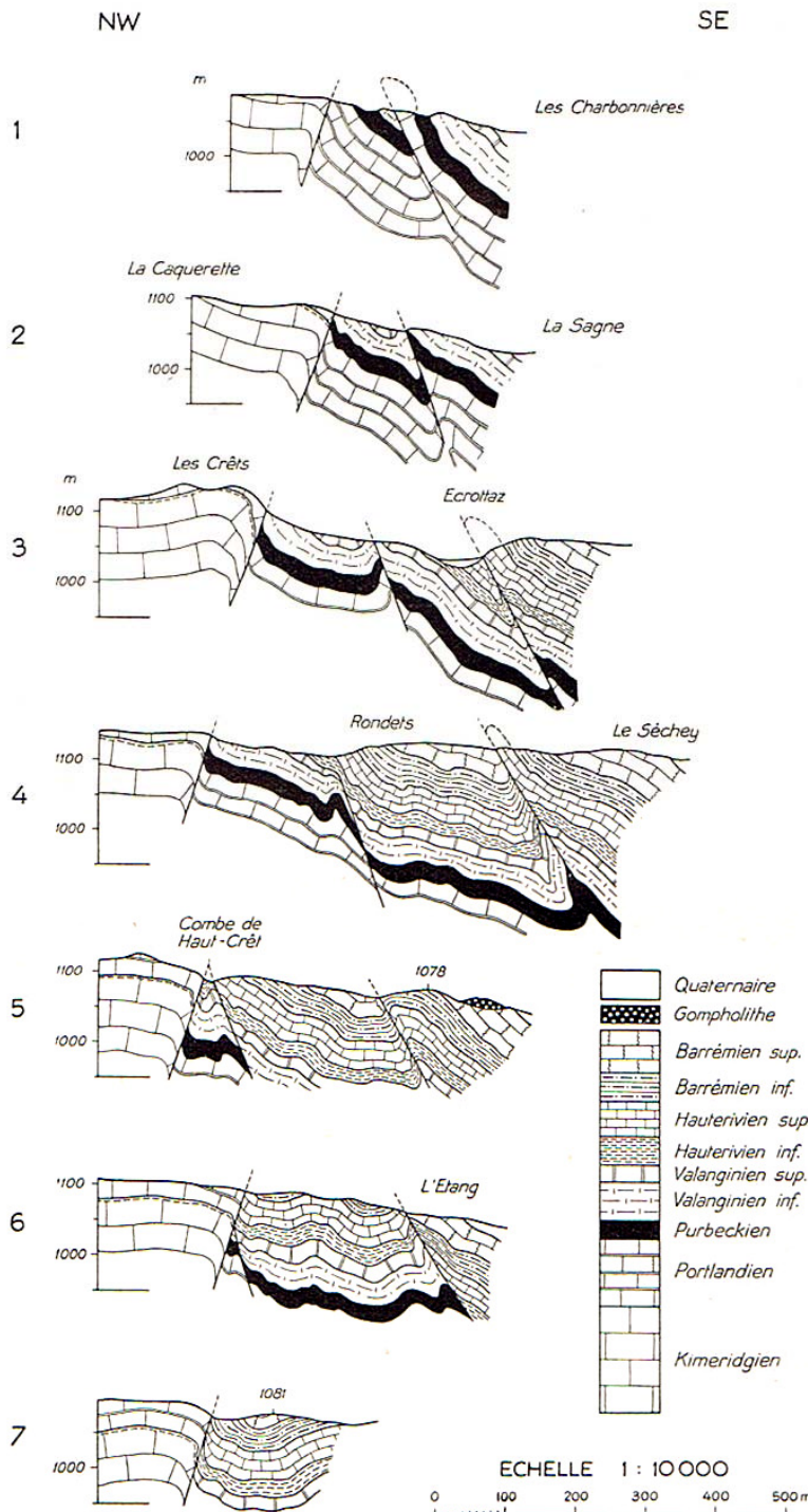
Fig. 19. Coupes tectoniques entre les Charbonnières et le Lieu.
