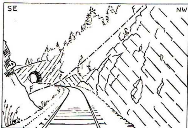
Fig. 18. L'enjambement de Pré Lionnet (Le Lieu).
